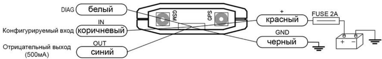
Расположение выводов модуля
